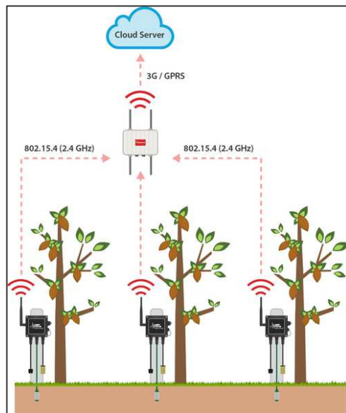
Collecte d'information grâce aux capteurs au sol
